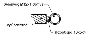
ΛΕΠΤΟΜΕΡΕΙΑ ΠΟΝΤΑΡΙΣΜΑΤΟΣ ΣΩΛΗΝΑ Ø12x1mm
