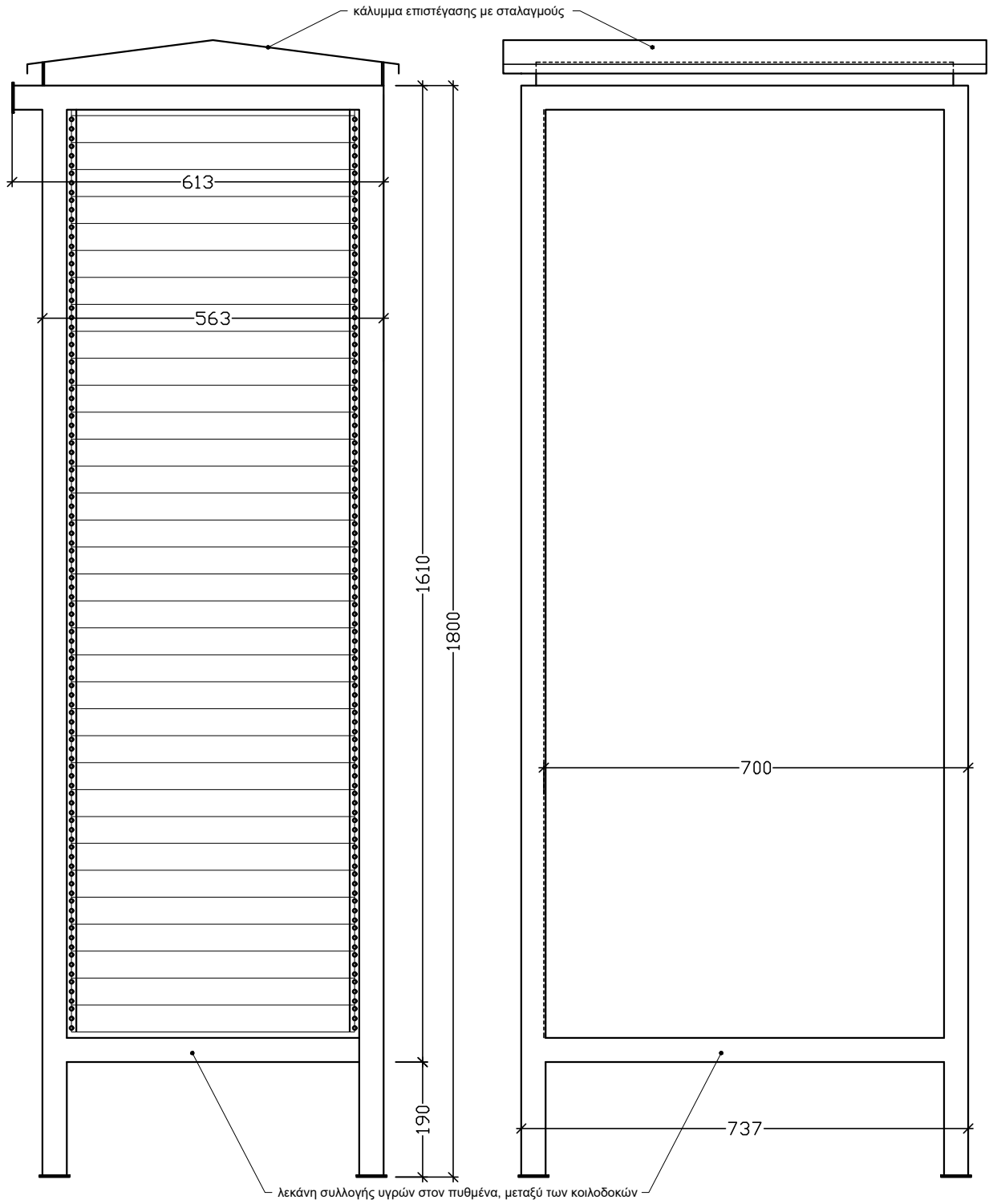
ΠΡΟΣΘΙΑ ΟΨΗ
