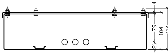
ΛΕΠΤΟΜΕΡΕΙΑ ΠΟΝΤΑΡΙΣΜΑΤΟΣ ΣΩΛΗΝΑ Ø12x1mm
