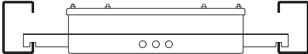
ΛΕΠΤΟΜΕΡΕΙΑ ΠΟΝΤΑΡΙΣΜΑΤΟΣ ΣΩΛΗΝΑ Ø12x1mm
