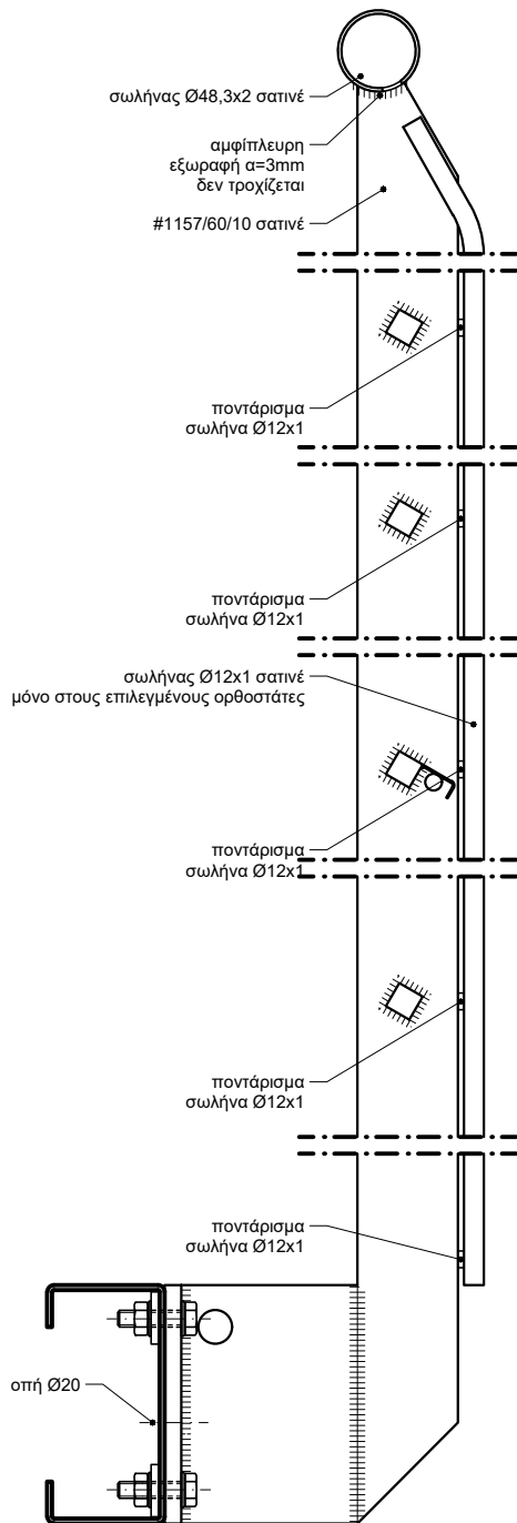
ΤΡΟΠΟΣ ΤΟΠΟΘΕΤΗΣΗΣ ΣΩΛΗΝΑ ΚΑΛΩΔΙΩΝ
