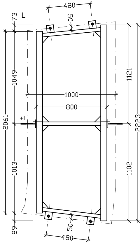
П 2.17 \begin{matrix} \Gamma & 44,6 \\ & 51,4 \end{matrix}
