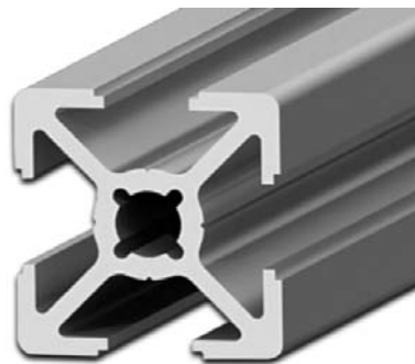
Προφίλ γενικών κατασκευών
