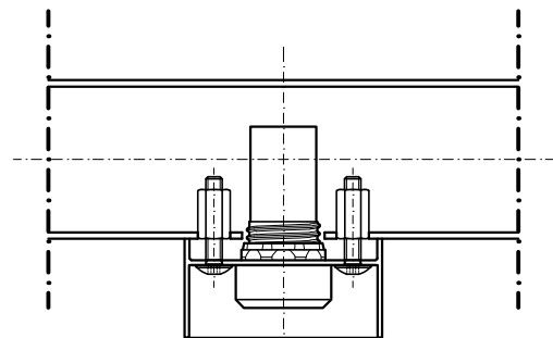
ΤΟΜΗ ΔΙΑΜΗΚΗΣ
