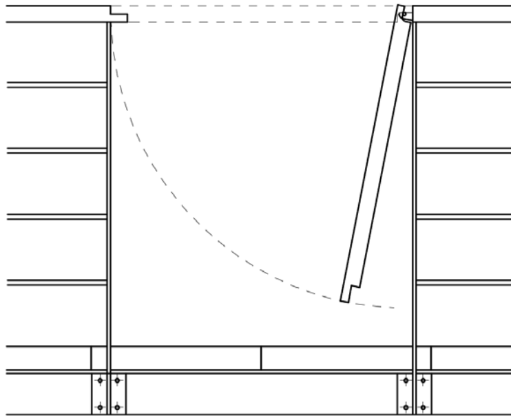
Τυπική μορφή θύρας κιγκλιωμάτων σε όψη.
